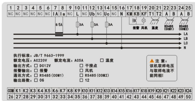
PEF2100, 2200 系列功控器接线示意图
